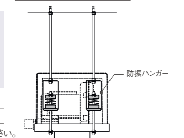
エアブローポンプ天井吊り施工例
